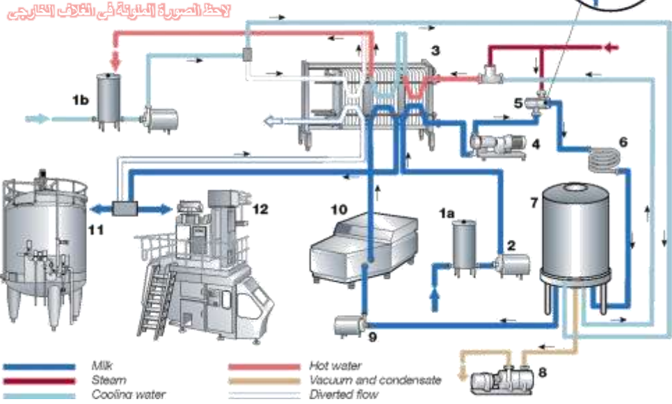
الشكل رقم (204) المعاملة بالحرارة الفائقة UHT بأسلوب حقن البخار في المنتج، عن (Bylund, 1995).
