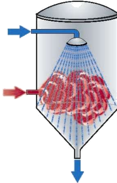
الشكل رقم (205) يوضح عملية رش الحليب في جو من البخار Infusion، عن (Bylund, 1995).
