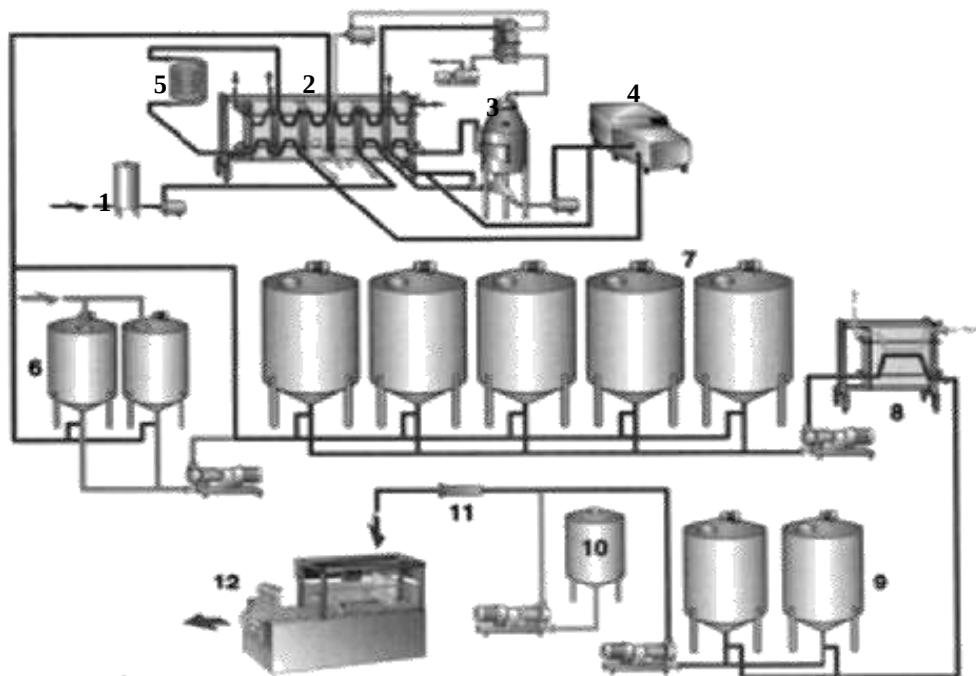
(1) حوض الموازنة، (2) المبادل الحراري، (3) المبخر، (4) المجنس، (5) أنبوب الحجز، (6) خزانات بادئ التصنيع، (7) خزانات التخمر، (8) مبرد صفانحي، (9) خزانات حجز، (10) خزان النكهة، (11) وحدة مزج الزبادي مع النكهة، (12) ماكينة التعبئة.
