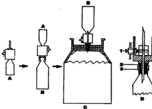
(A) مزرعة البائى الأم (B) مزرعة البائى الوسطي (C) بائى التصنيع (D) تركيب تفصيلي للإبرة: (1) صنبور (2) لحام معدني (3) محلول هيبوكلوريت الصوديوم
