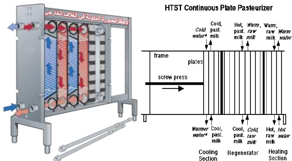
الشكل رقم (196) وضعية الصفائح وطريقة مرور الحليب وسوائل التسخين والتبريد بينها في جهاز البسترة السريعة، (يمين) عن (Goff, 2008)، (يسار) عن (Bylund, 1995).
