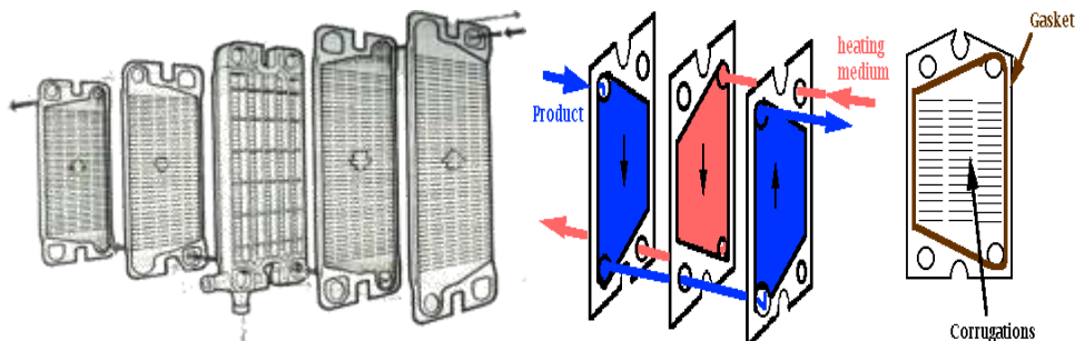
الشكل رقم (195) يوضح شكل المسخنات الصفانحية Plate Heaters وطريقة مرور الحليب بينها، (يمين)
