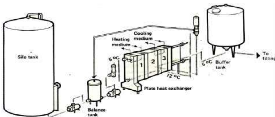
الشكل رقم (194) يوضح عملية البسترة التي تجرى للحليب السائل بواسطة جهاز البسترة السريعة، عن (Bylund, 1995).
